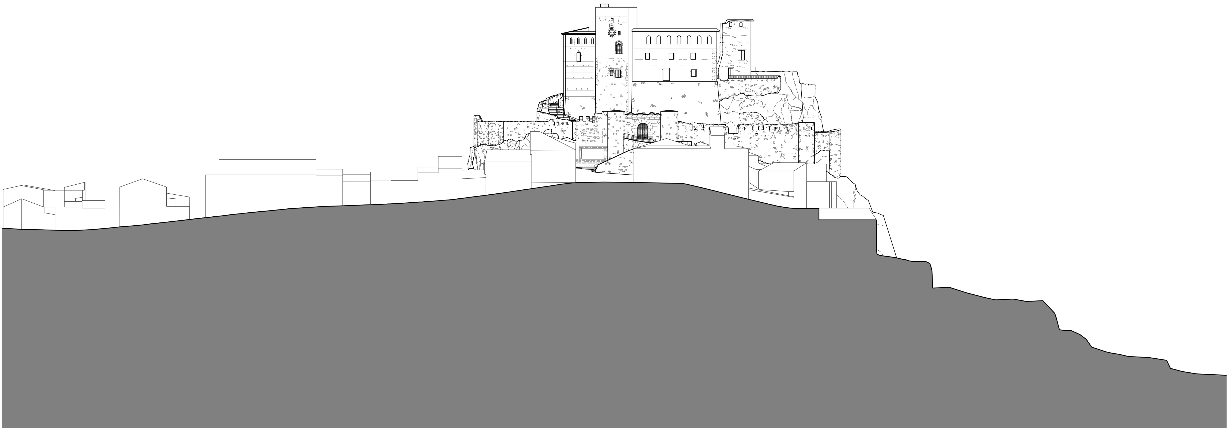
SECCIÓN SUR-NORTE, POR CALLE GENERAL PRIM Y CALLE LAVADERO
